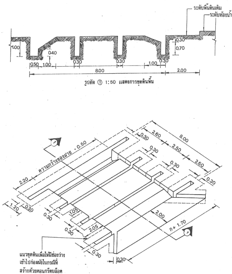
รายละเอียดการเตรียมที่และขุดดิน
