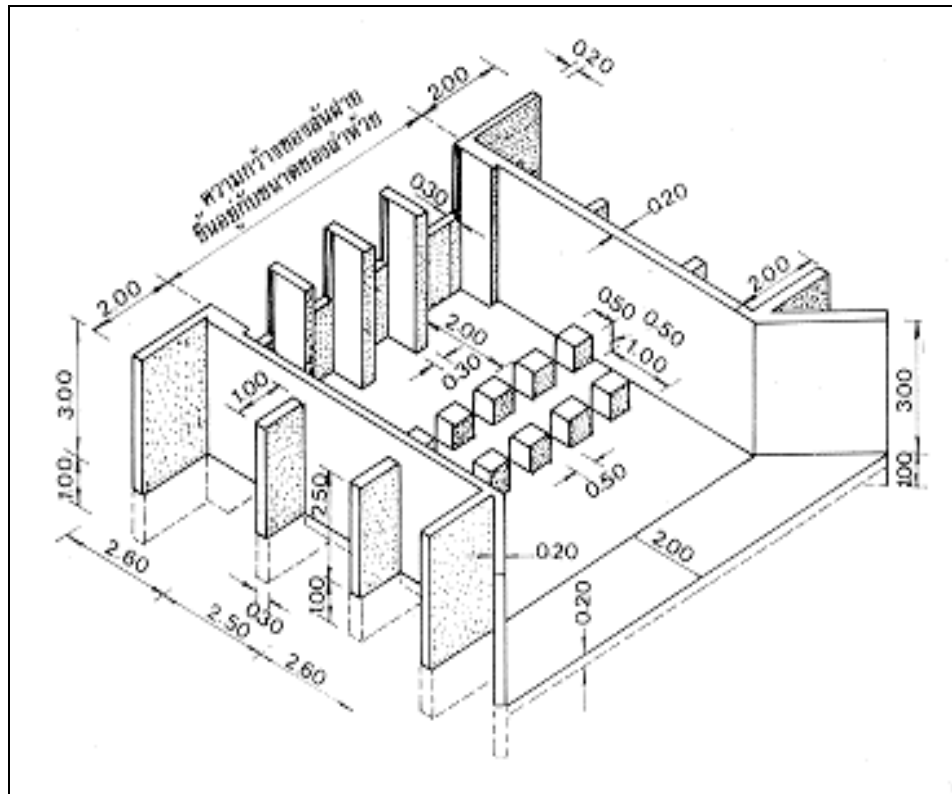
รูปที่ 5.11 แบบมาตรฐานฝ่าย ม.ร.ร. 2527 ที่มีส้นฝ่ายสูง 1.50 เมตร ผนังข้างสูง 3.00 เมตร
