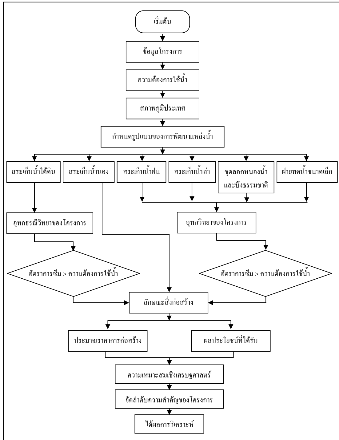
รูปที่ 3.1 แสดงแผนภูมิการศึกษาความเหมาะสม โครงการสระเก็บน้ำ ชุดลอกหนองน้ำ และบึงธรรมชาติและฝายทดน้ำขนาดเล็ก
