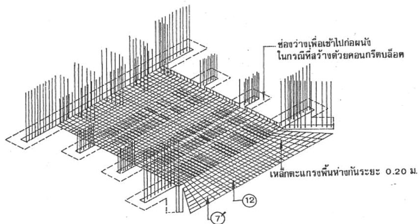
แบบแสดงการวางเหล็กพื้น
