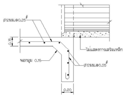
รูปขยาย ③ มาตราส่วน 1:25
