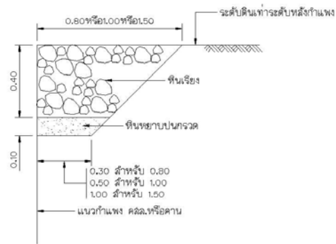
ขยายหินเรียง ② สำหรับกว้าง 0.80, 1.00 และ 1.50 ม. มาตราส่วน 1:20
