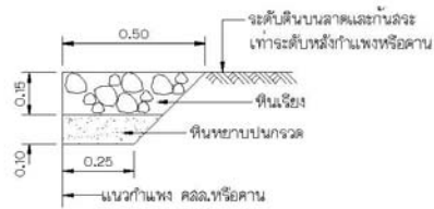
ขยายหินเรียง ① สำหรับกว้าง 0.50 ม. มาตราส่วน 1:20
